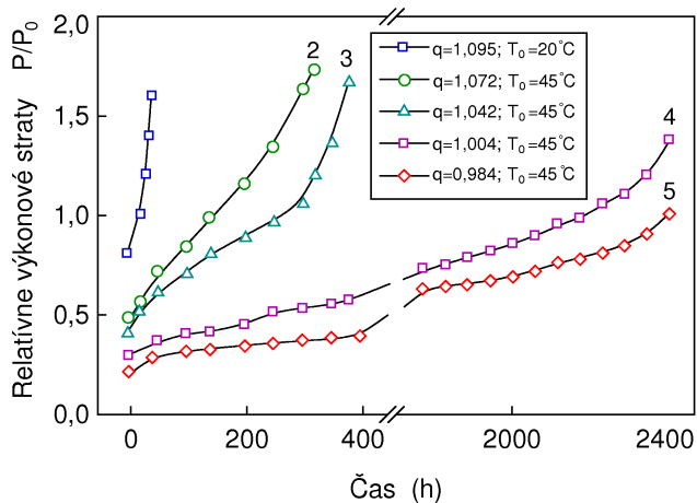
Obr. 2. Závislosť výkonových strát pri rôznych priložených napätiach a teplotách [11]
